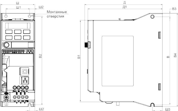
Рисунок 1 – Габаритные и присоединительные размеры прибора типоразмеры 1 и 2
