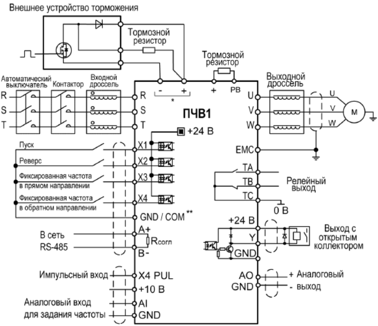
Рисунок 7 – Общая схема подключения
