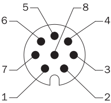
Вид разъема устройства M12 со стороны кабеля / устройства
